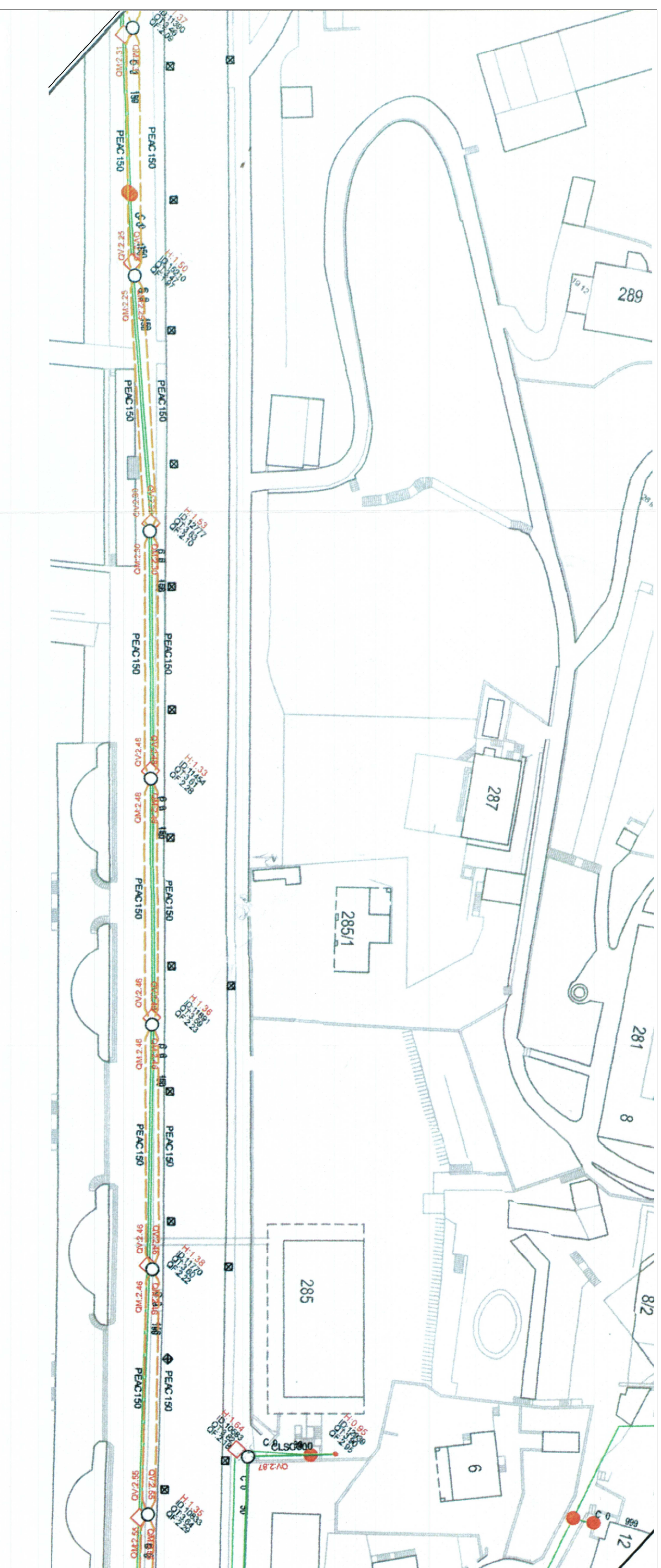
MAPPA ACEGAS - CANALI FOGNATURE scala 1:500
