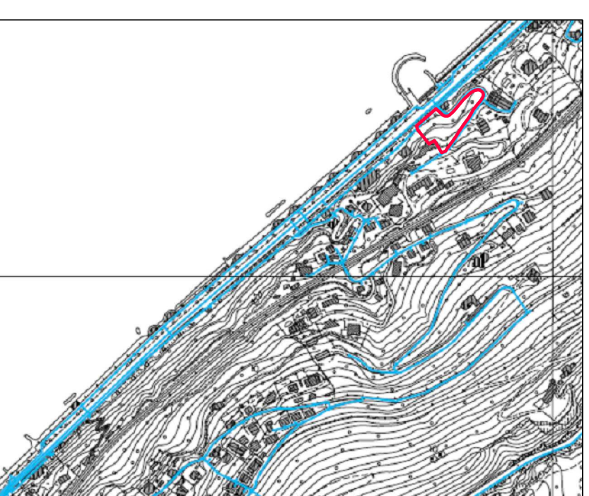
ESTRATTO P.R.G.C. Rete idrica - scala 1:10000
