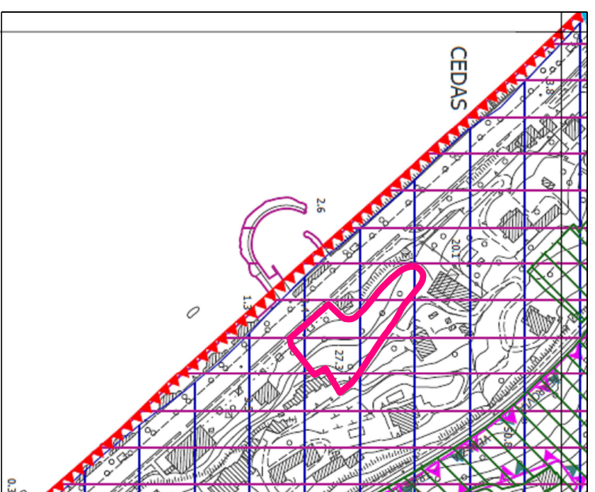
ESTRATTO P.R.G.C. Vincoli - scala 1:5000
